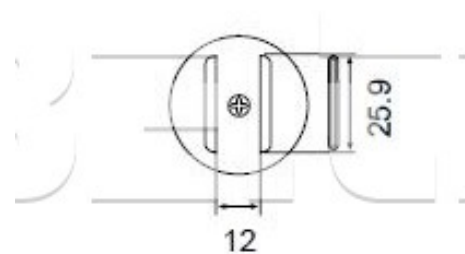
A1214B SOJ 10 x 26
