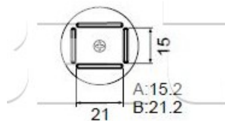
A1128B QFP 14 x 20
