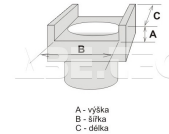
Rozměry jsou v milimetrech, kromě délky pro rozměr C, která je uvedena v záhlaví Popisu.
